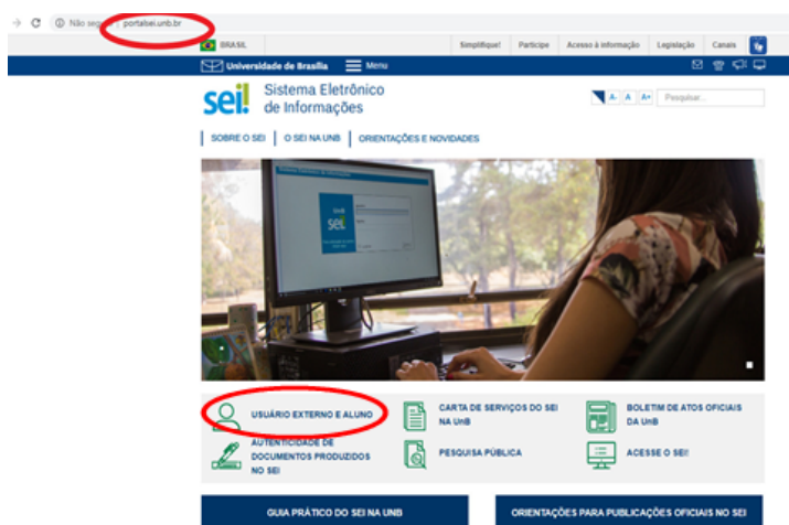
Figura 2: Portal SEI
